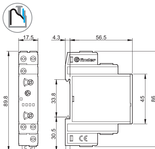
Tipo 80.51 Morsetti Push-in
