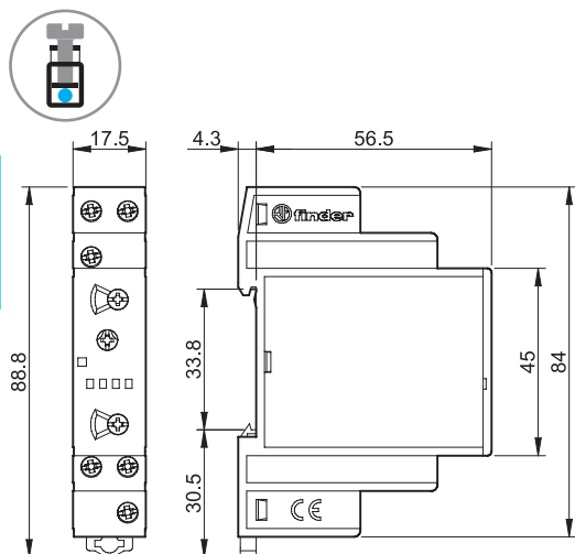
Tipo 80.51 Morsetti a vite
